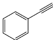
Molecule 4
